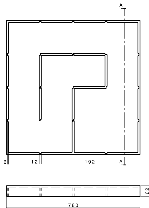
Corte A-A
